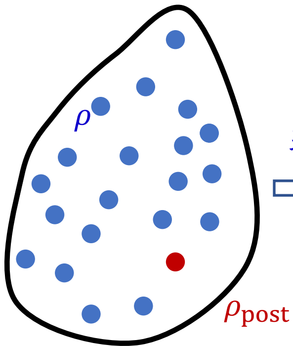
概率密度空间 \mathcal{P}
