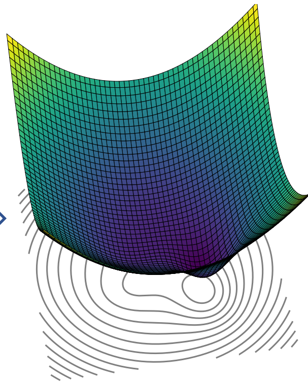
度量空间 (\mathcal{P}, M(\rho))
