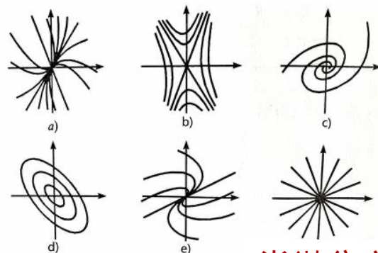
常微分方程
